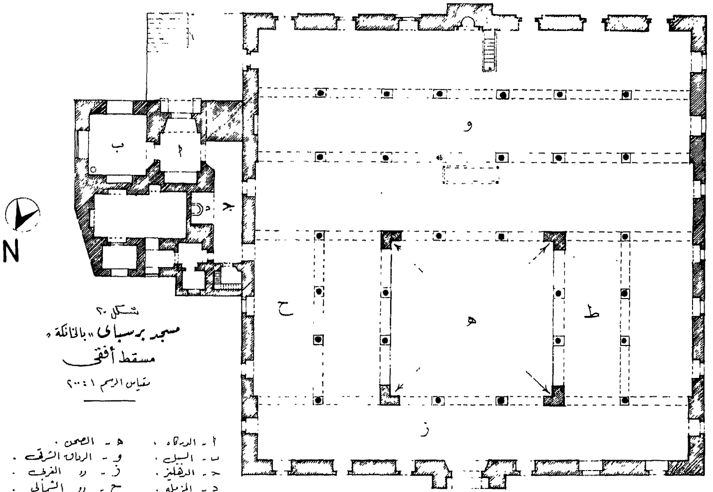
شکل ( ۷ ) یبین مستطافق لجامع الاشراف برسبای بالخانه بمحافظة القلیوبیة
